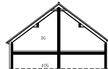
SCHNITT ZWERCHGIEBEL GARTENSEITE HAUS A
