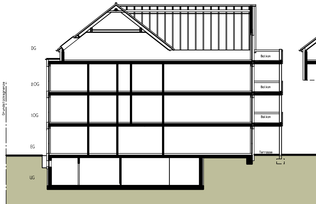
SCHNITT 1 - 1 HAUS A
